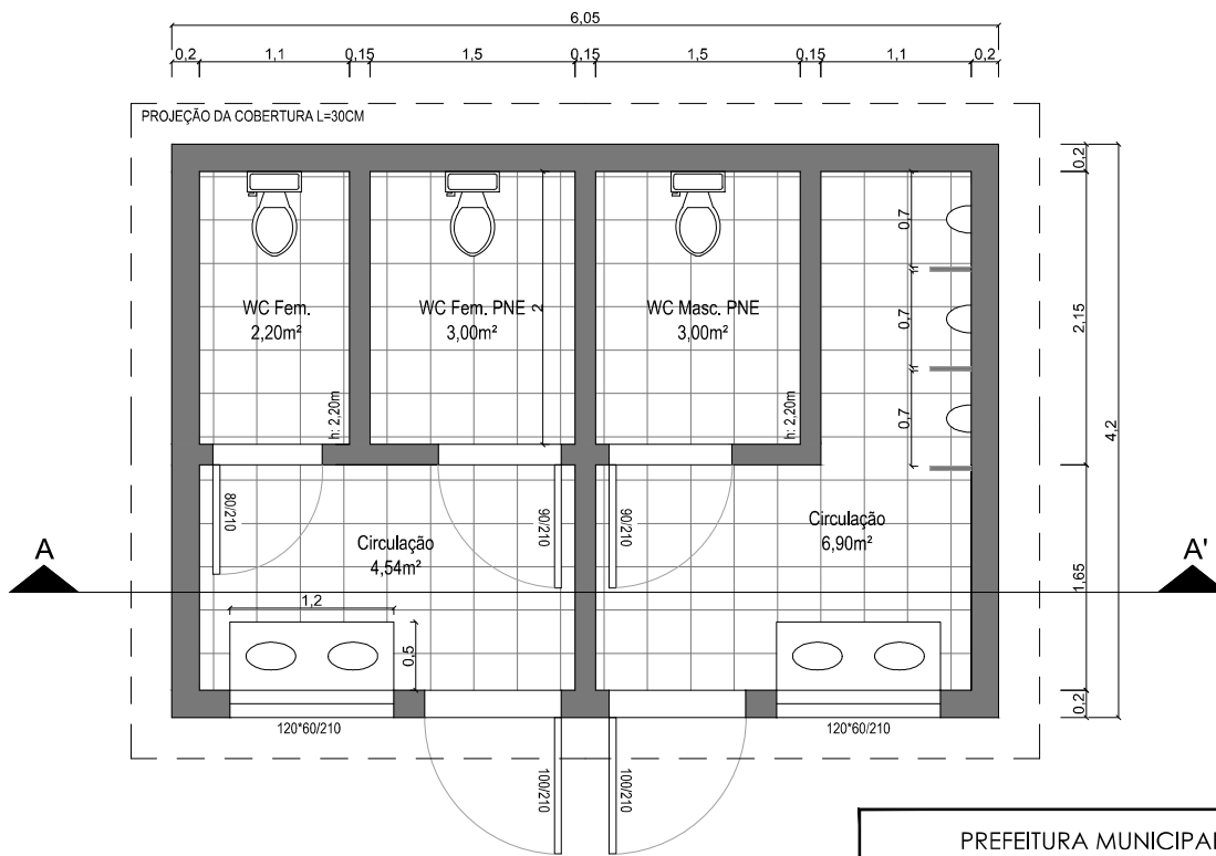
1 PLANTA BAIXA
