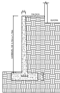
1 CORTE A-A'
